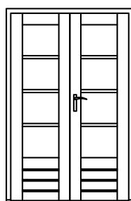
WM02H 1210 X 1935 mm (Milchglas)
