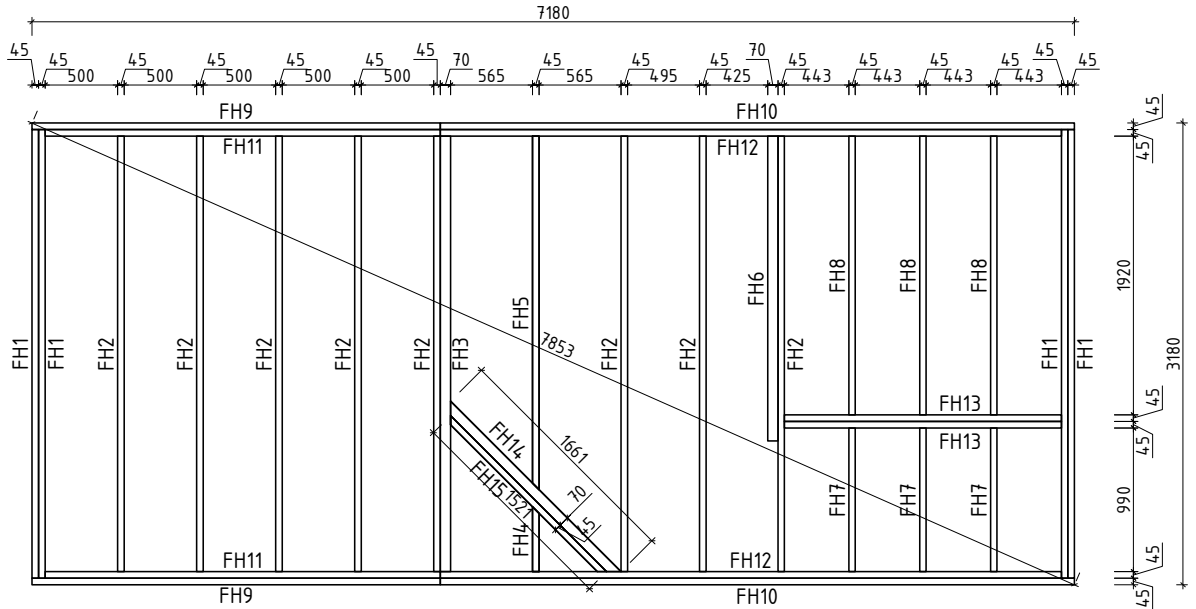
Fundamentplan für Aufbau Terrasse links
