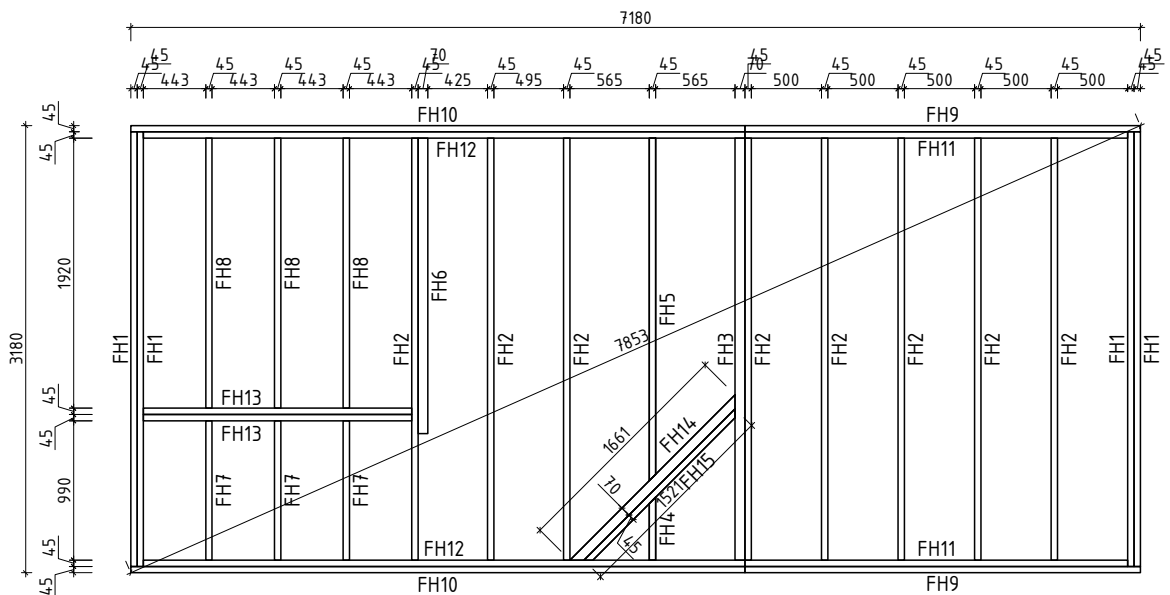
Fundamentplan für Aufbau Terrasse rechts
